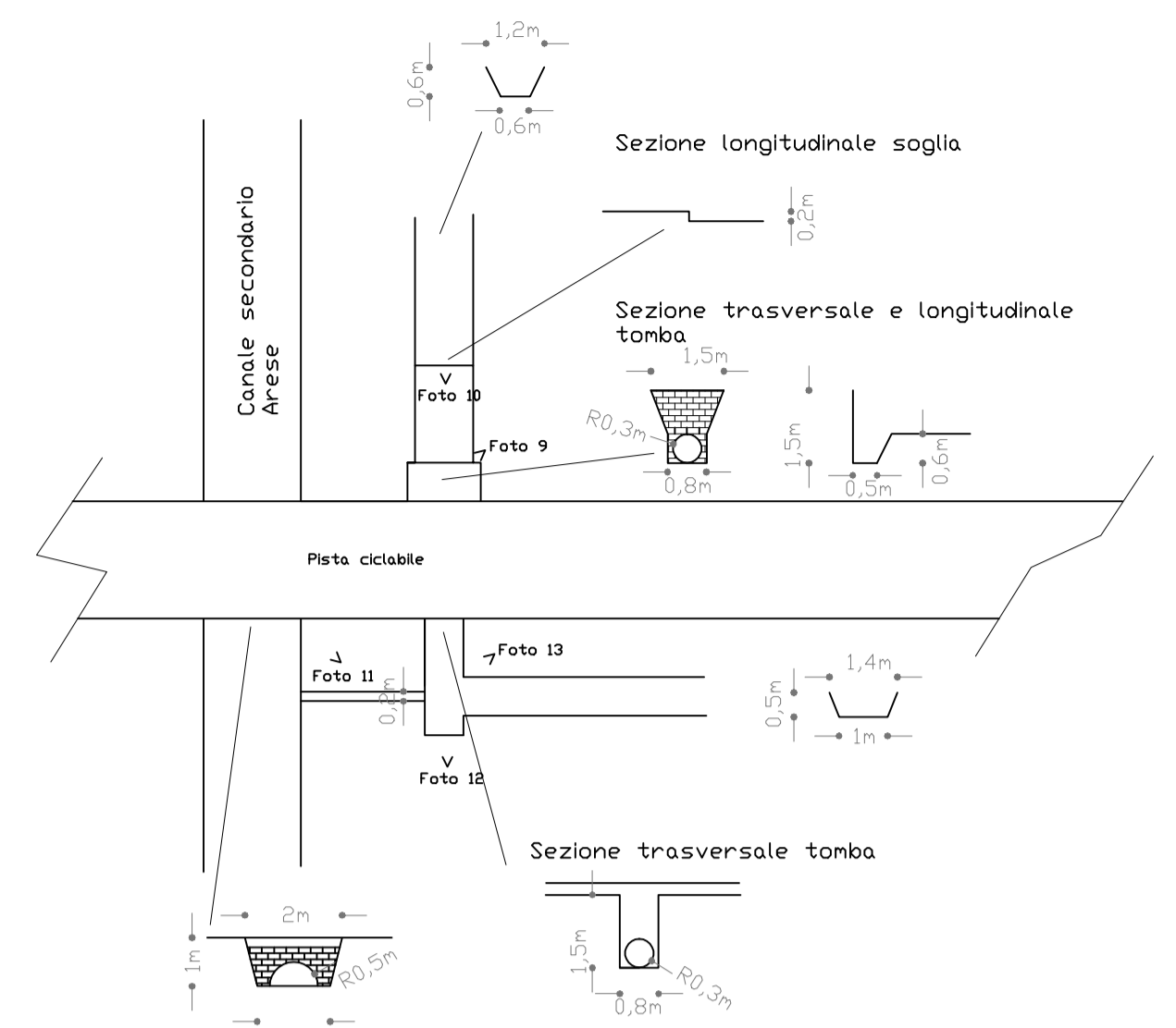
Sezione longitudinale soglia
