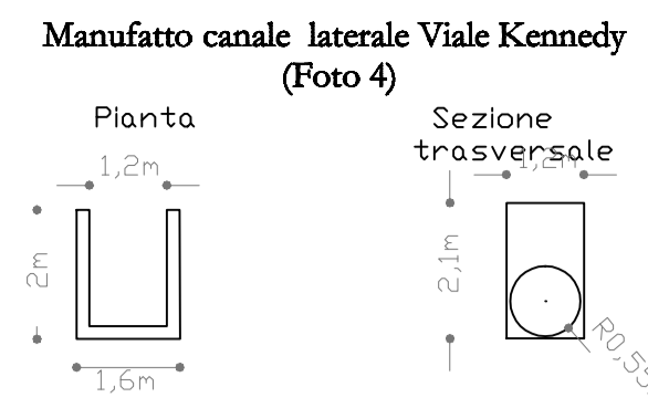
Manufatto canale laterale Viale Kennedy (Foto 4)
