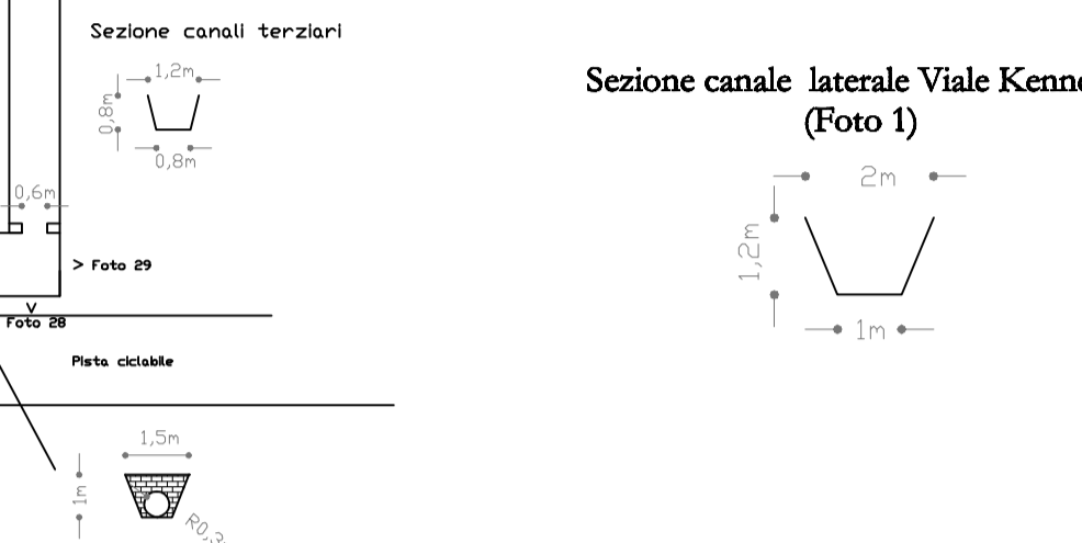
Sezione canale laterale Viale Kennedy (Foto 1)
